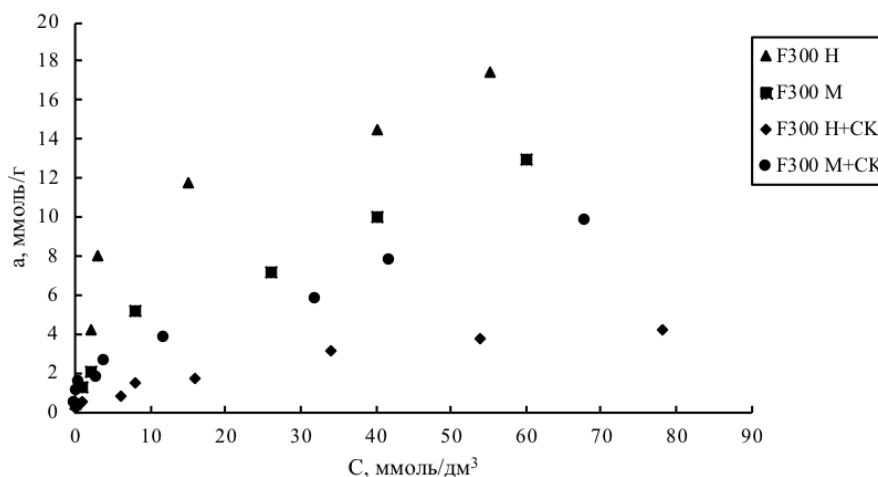
Рисунок 2 – Изотермы адсорбции меди на F 300 Н и F 300 М из растворов \text{CuSO}_4 без СК и в присутствии сульфаниловой кислоты
