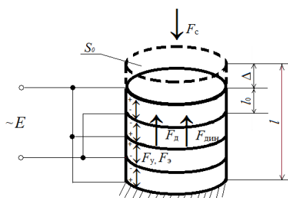
Рисунок 1 – Конструкция наборного столба пьезоэлектрических шайб с продольной поляризацией
