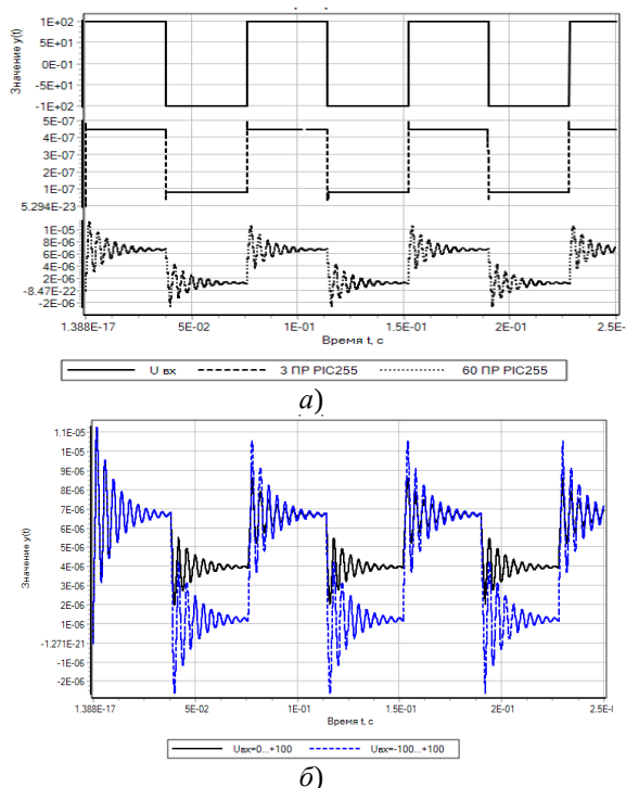
Рисунок 7 – Исследование перемещения наборных столбов при однополюсном (а) и двухполюсном (б) напряжении сигнала управления
