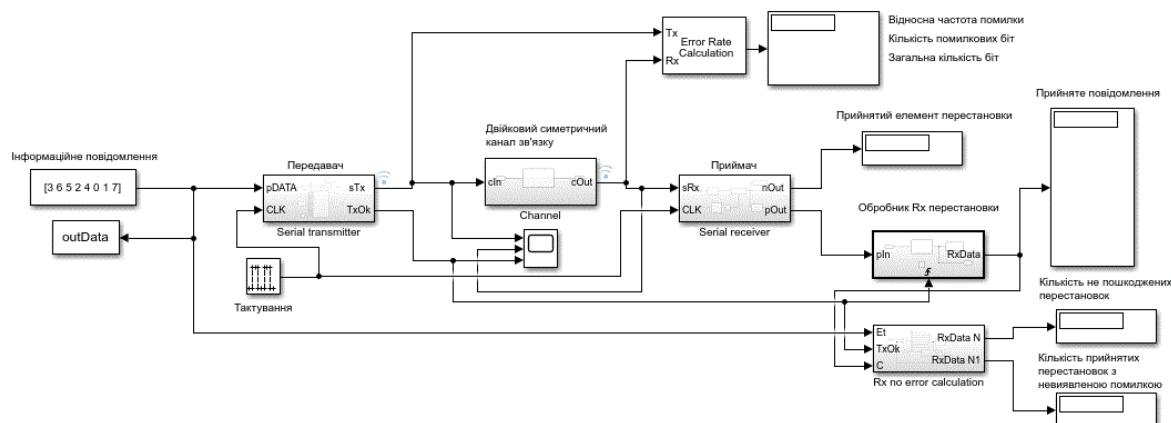
Рисунок 2. Модель системи передавання перестановки каналом зв'язку
