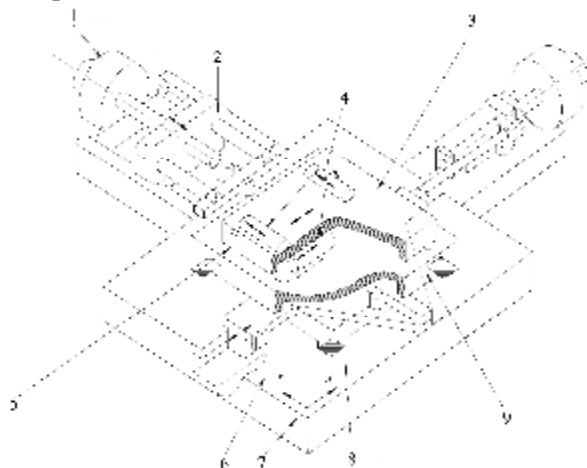
Рис. 2. Схема системы экспонирования в разрезе: 1 – двигатель постоянного тока; 2 – рама привода оси Y; 3 – платформа прецизионного перемещения; 4 – пьезоэлектрический актуатор; 5 – поддерживающий гибкий вал; 6 – плоскость перемещения XY; 7 – основание; 8 – слайдер; 9 – столик грубого перемещения
