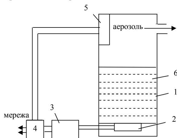
Рис. 1. Схема небулайзера: 1 – корпус; 2 – п'єзоелектричний перетворювач; 3 – електрична схема; 4 – адаптер; 5 – вентиль; 6 – рідина, яка розпилюється
