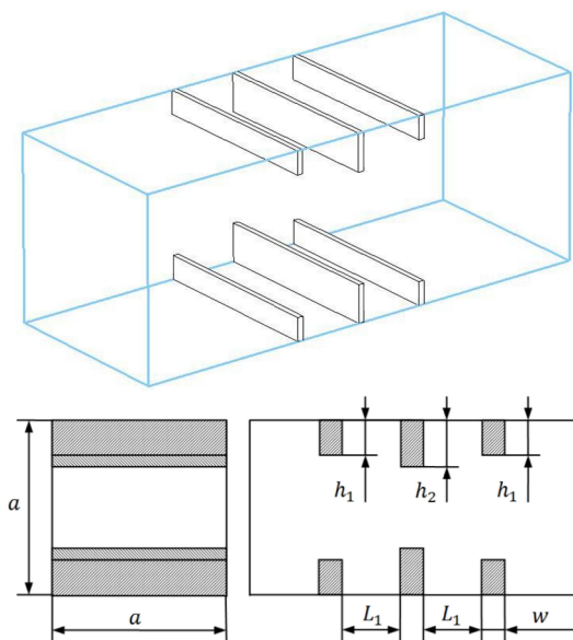
Рисунок 1 – Трехмерная модель квадратного волновода поляризатора с тремя диафрагмами
