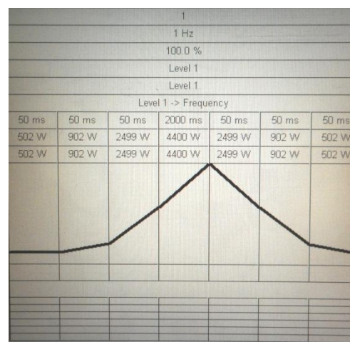
Рисунок 14 – Циклограма програми управління потужністю лазерного випромінювання при зварюванні за режимом № 1331.2
